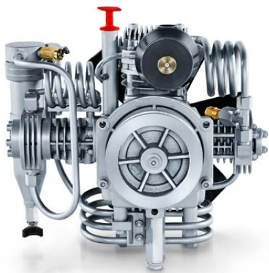
Kompressorblock PE 100
